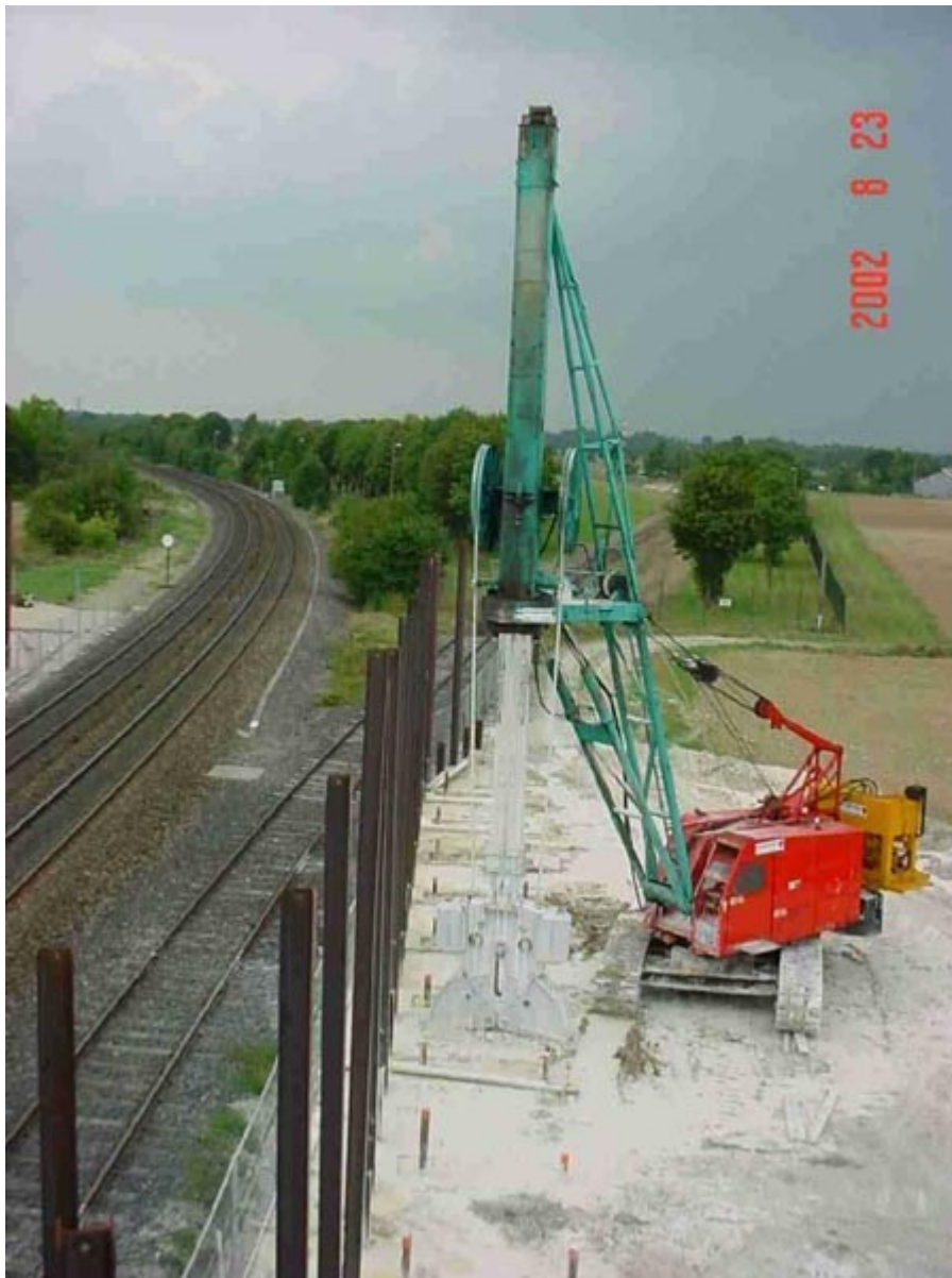
Forage des barettes pour un pont-rail (Photo FNTF)
